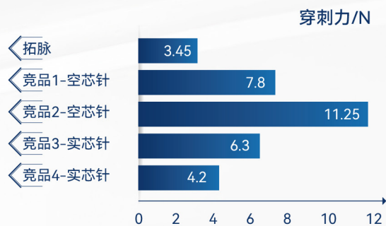
模拟穿刺穿刺力对比
