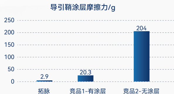
导引鞘涂层摩擦力测试数值对比
